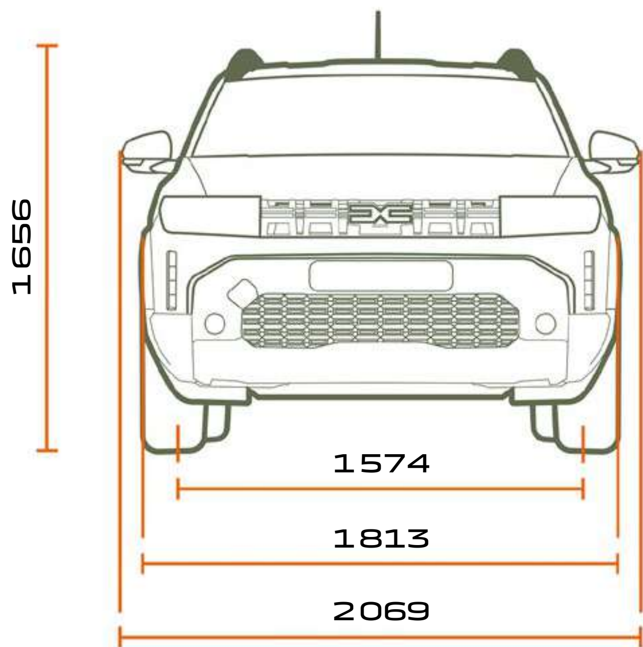
VUE AVANT
