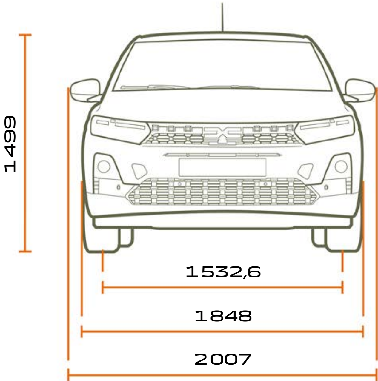
VUE AVANT
