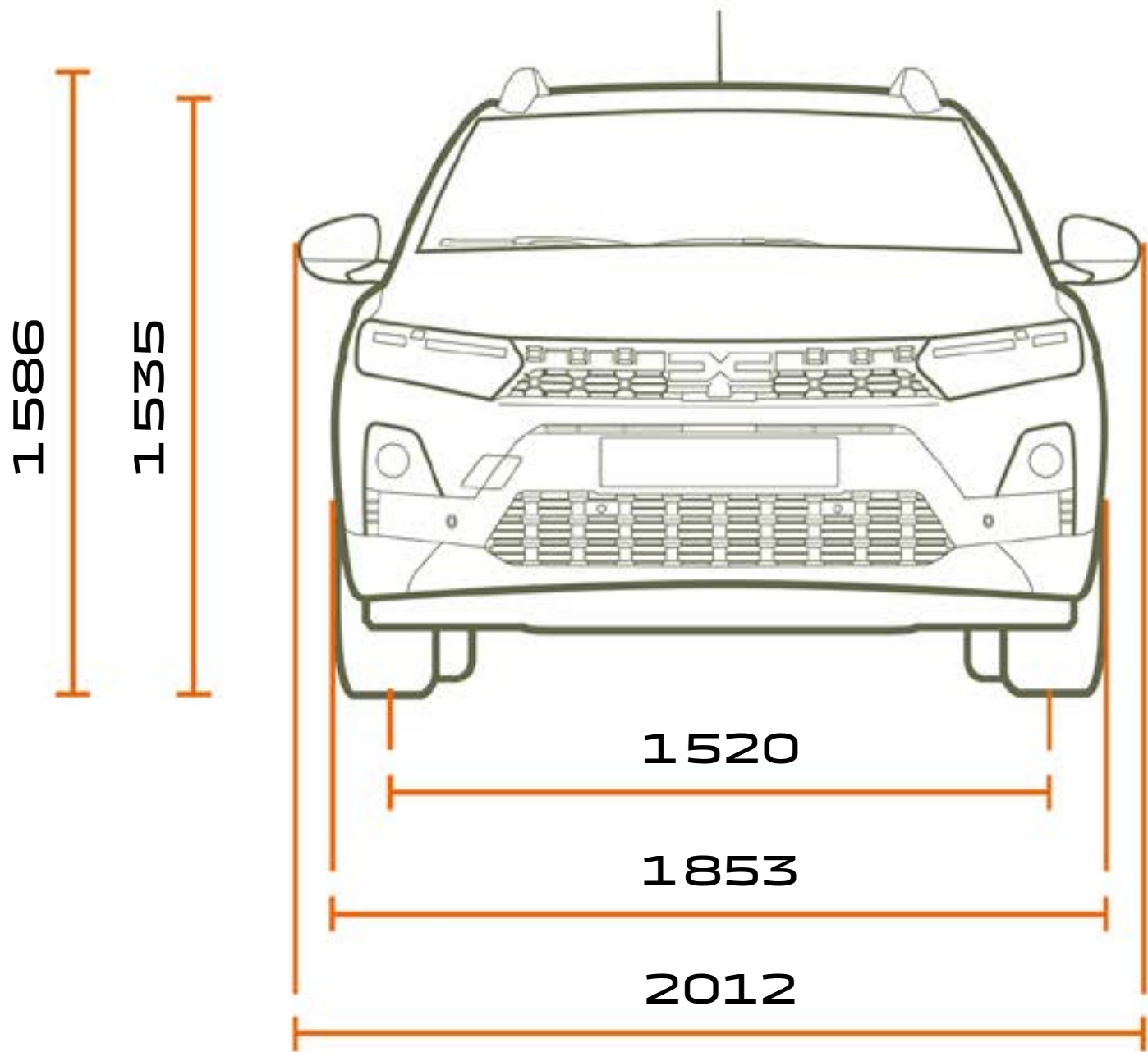
VUE AVANT
